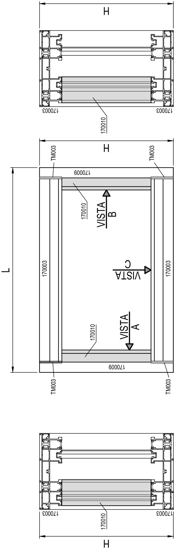
VISTA B
