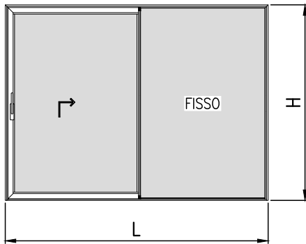
VISTA INTERNA
