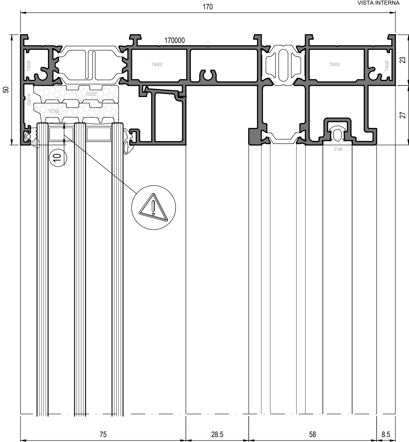
VISTA INTERNA
