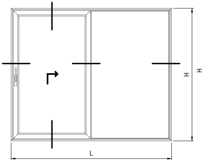
PROSPETTO INTERNO
