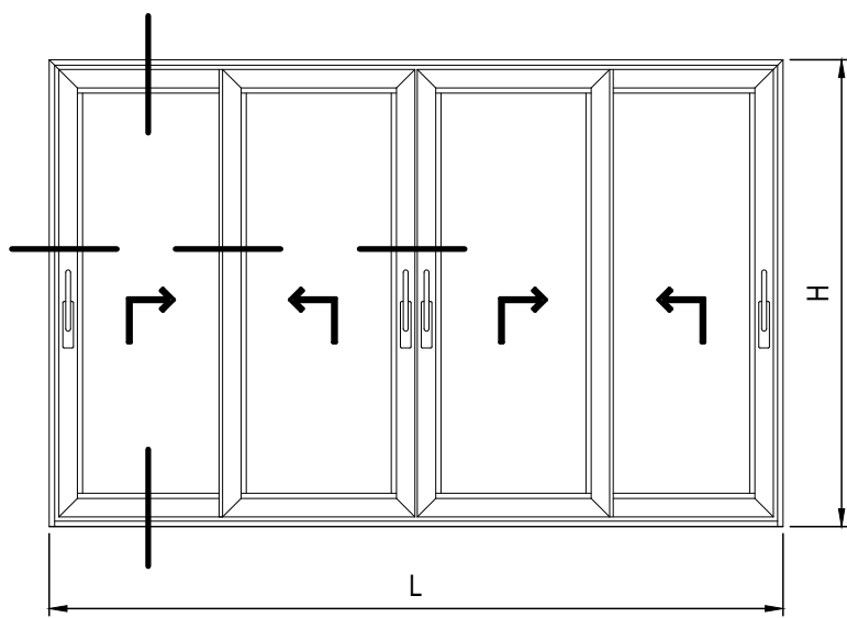
PROSPETTO INTERNO
