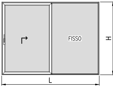
VISTA INTERNA
