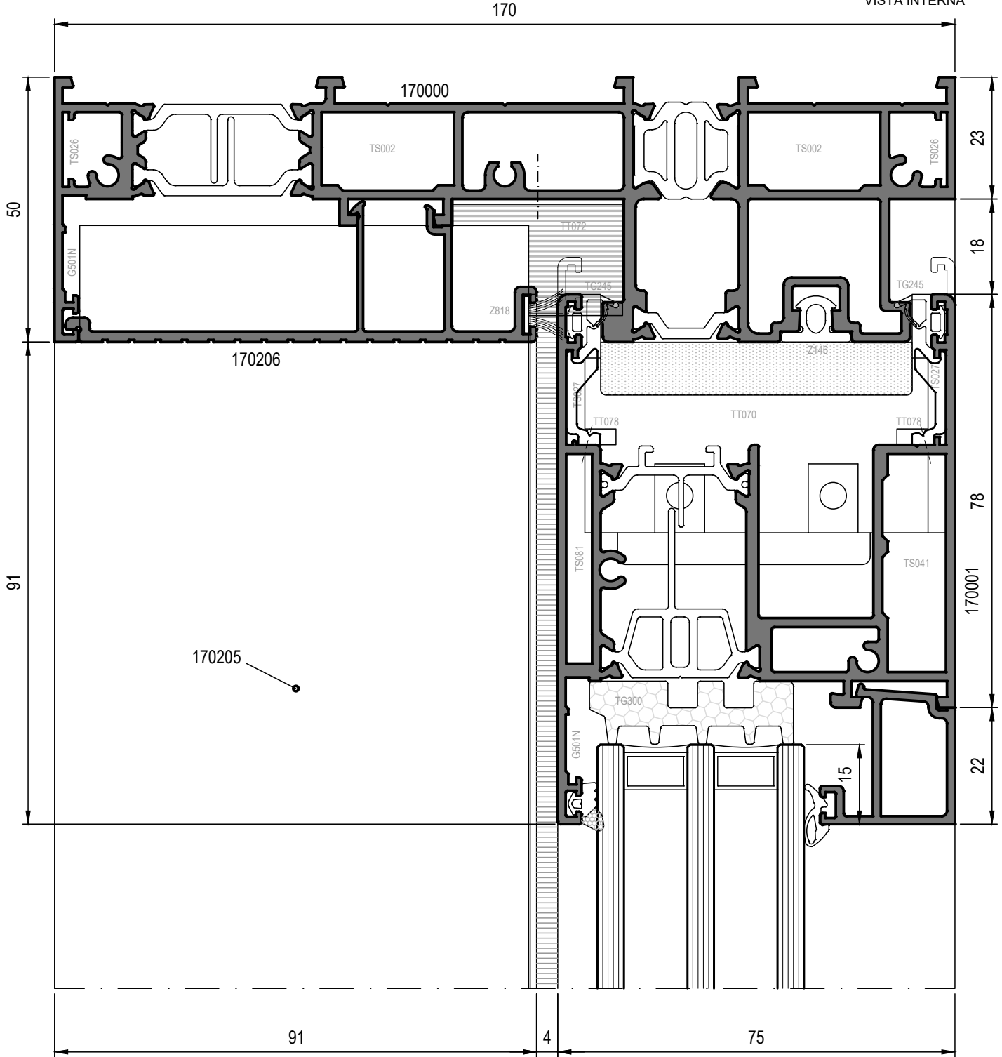
VISTA INTERNA
